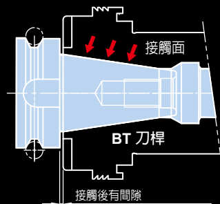
單面接觸主軸型式
