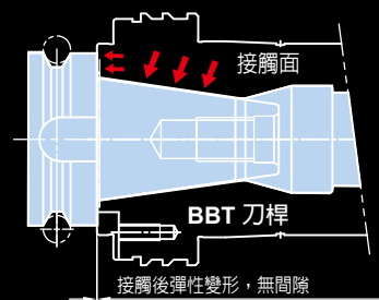
雙面接觸主軸型式
