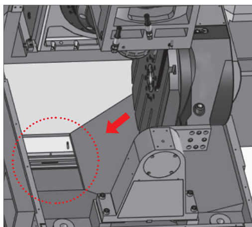
底座落屑口設計
